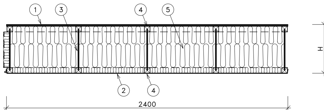
Figur b Tvärsektion
